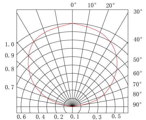
图.6 辐射特性曲线
