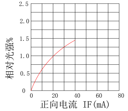
图.4 正向电流与相对光强曲线
